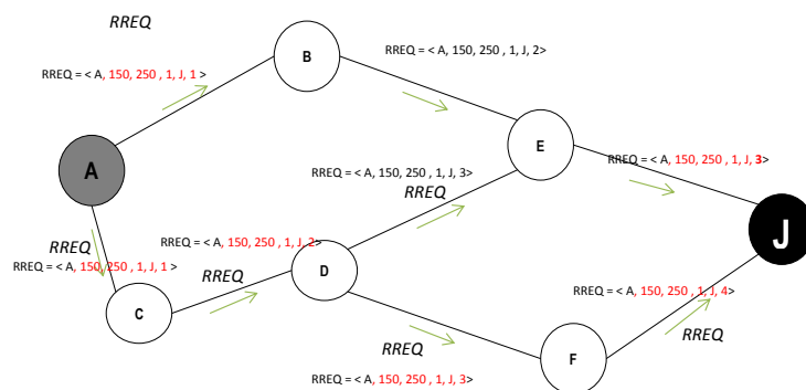
FIGURE 2.6 – Exemple d'illustration de l'algorithme de routage à la demande AODV
