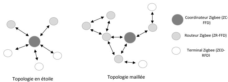
FIGURE 2.5 – topologies du réseau ZigBee
