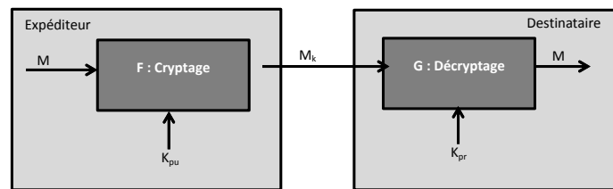
FIGURE 1.12 – Principe du cryptage asymétrique
