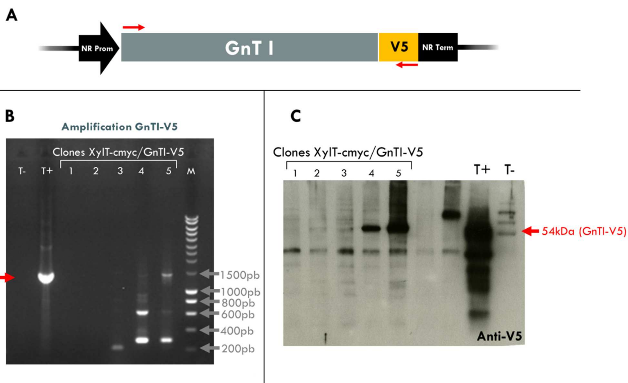
Figure 85 : Criblage des co-transformants GnT I-V5 et XylIT-cmyc par PCR et western-blot
