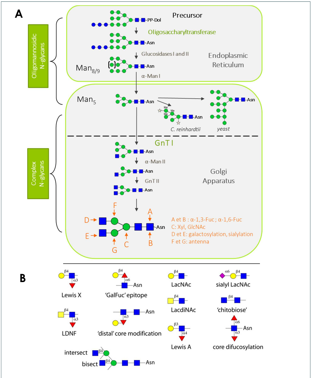
Figure 29 : Biosynthèse et maturation des N-glycannes dans le réticulum endoplasmique et l'appareil de Golgi.
