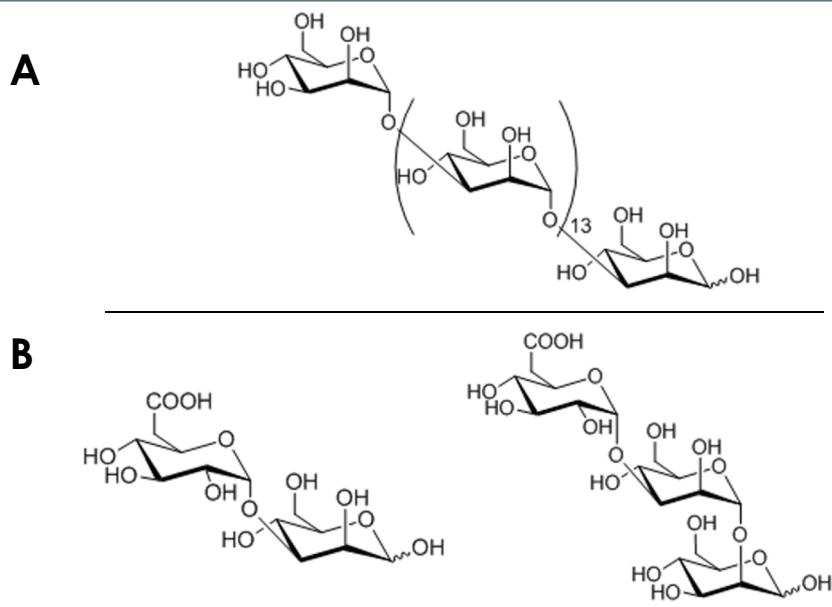
Figure 8 : Structure putative des polysaccharides pariétaux retrouvés chez P. tricornutum (Gügi et al., 2015).
