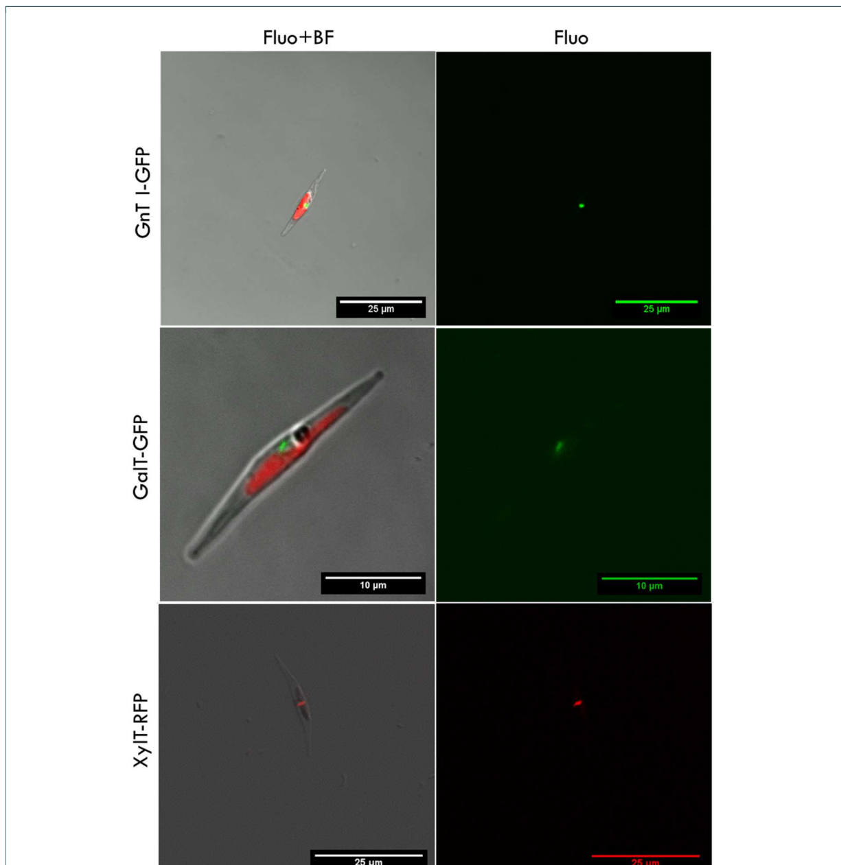
Figure 86 : Observation en microscopie confocale des cultures de P. tricornutum transfectées avec les constructions GnT I-GFP, GalT-GFP et XylT-RFP Le signal coloré en rouge pour les cellules GnT I-GFP et GalT-GFP correspond à l'autofluorescence plastidiale.
