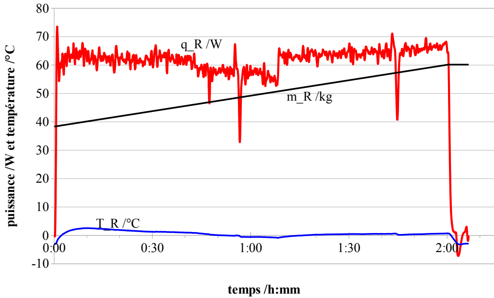
Illustration 17 : Ajout d'un équivalent d'acide nitrique sur l'aromatique.
