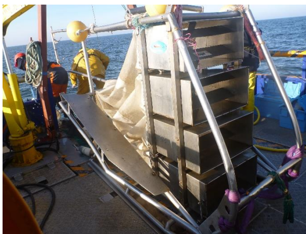
Figure 122 : Traîneau suprabenthique Macer-Giroq modifié (Dauvin & Lorgéré, 1989).
