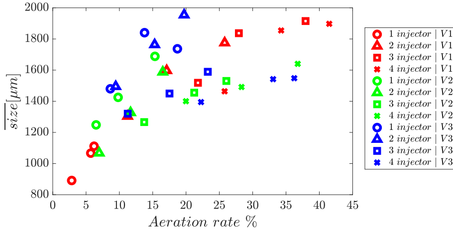
FIGURE 7 – Évolution de la taille moyenne des bulles en fonction du taux aération.
