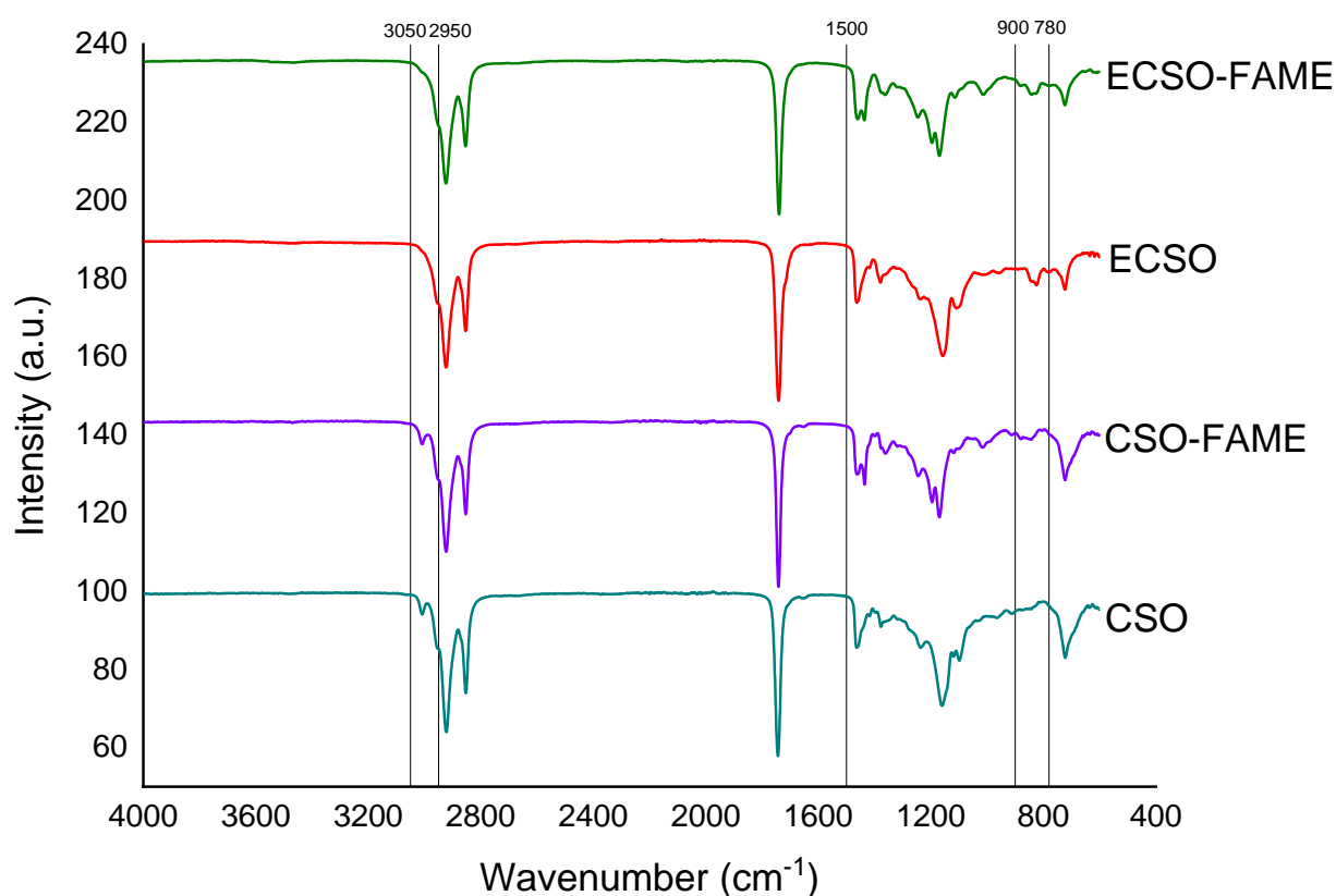
Figure 2. FTIR spectra for the CSO, CSO-FAME, ECSO and ECSO-FAME.
