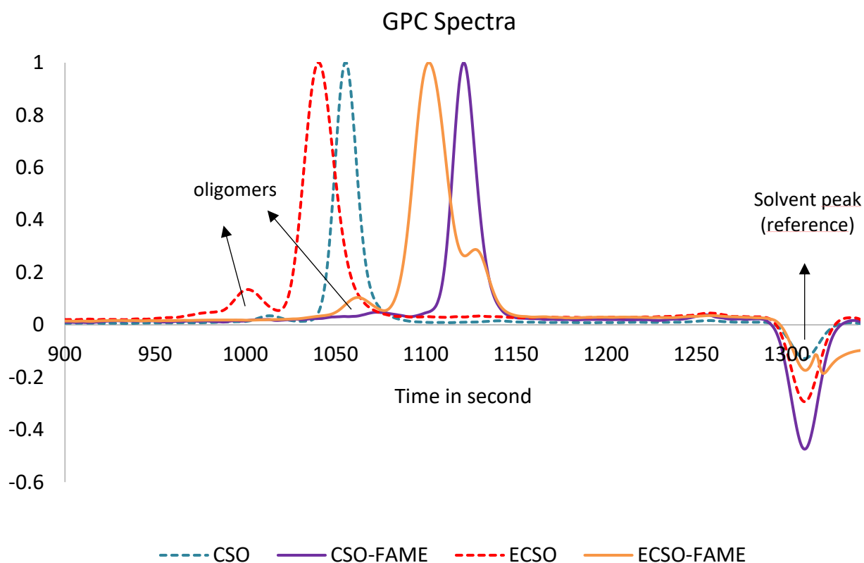
Figure 4. GPC spectra for CSO, CSO-FAME, ECSO and ECSO-FAME.
