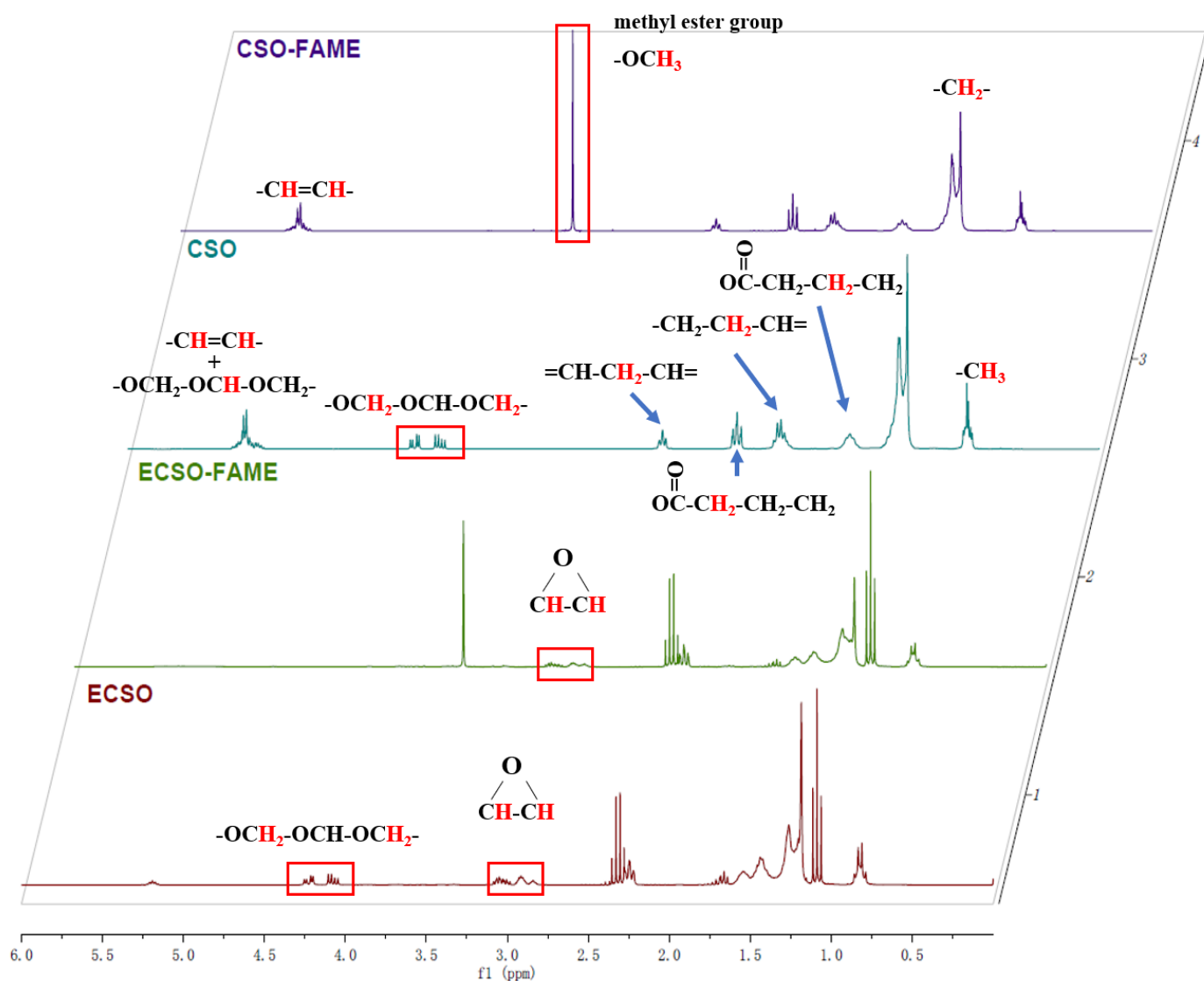
Figure 3. ^1\text{H} NMR spectra for CSO, CSO-FAME, ECSO and ECSO-FAME.
