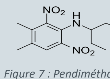
Figure 7 : Pendiméthaline
