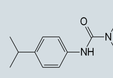
Figure 6 : Isoproturon
