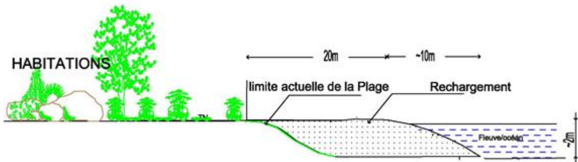
Figure 2. Schéma de l'engraissement de la plage de Pilote Bar (source : DEEC, 2015)
