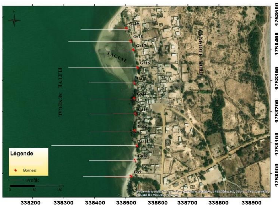
Figure 3. Localisation des profils topographiques
