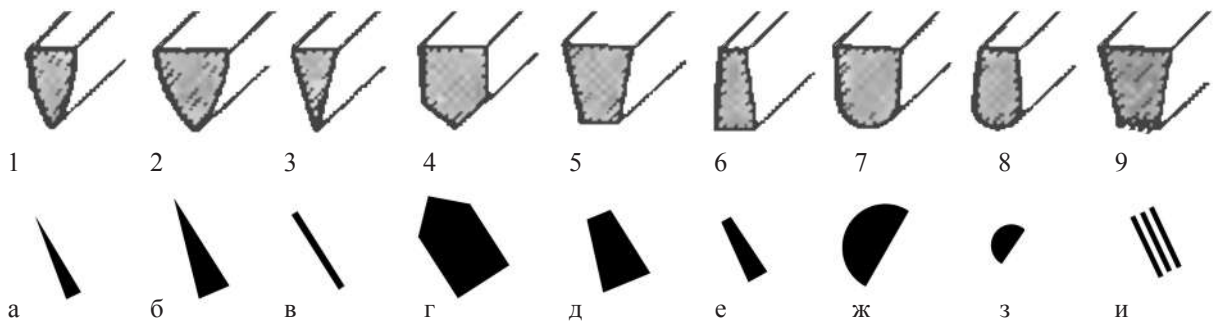
Рис. 1. Типы резцов (по: Бреполь 1982. Рис. 178) и их следы на изделиях: 1–2 – шпичштихель, узкий и широкий, 3 – мессерштихель, 4 – фасовочный штихель, 5–6 – фляхштихель, узкий и широкий, 7–8 – болштихель широкий и узкий; 9 – фанденштихель; а–б – равнобедренный треугольник, узкий и широкий, в – прямоугольник, г – пятиугольник с параллельными боковыми сторонами, д–е – трапеция, узкая и широкая, ж–з – полукруг большого и меньшего диаметра, и – ряды параллельных прямоугольников
