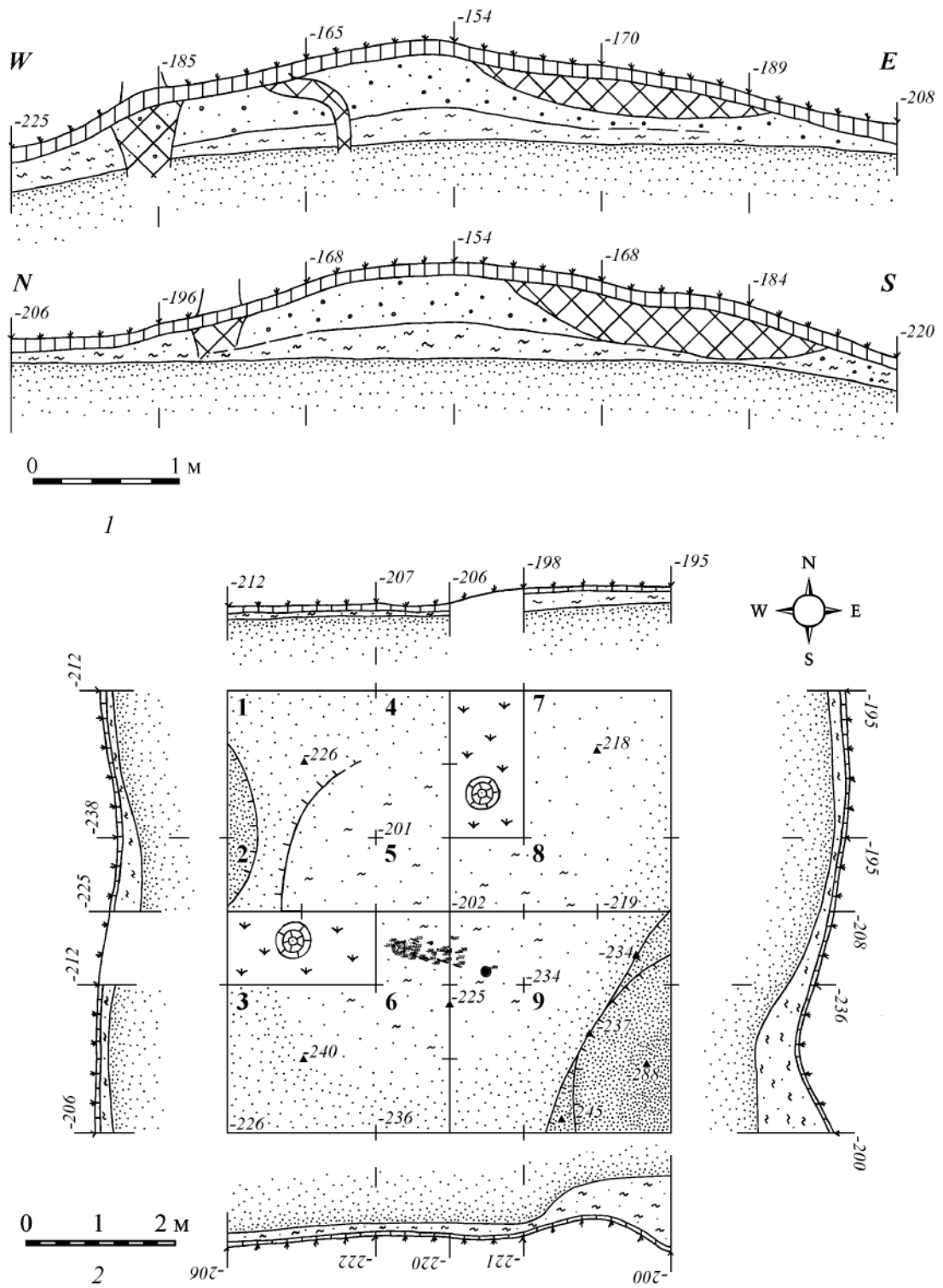
Рис. 2. Курганный могильник Навры. Курган 77: 1 – профили кургана; 2 – план кургана и профили раскопа. Рисунок Н. А. Плавинского
