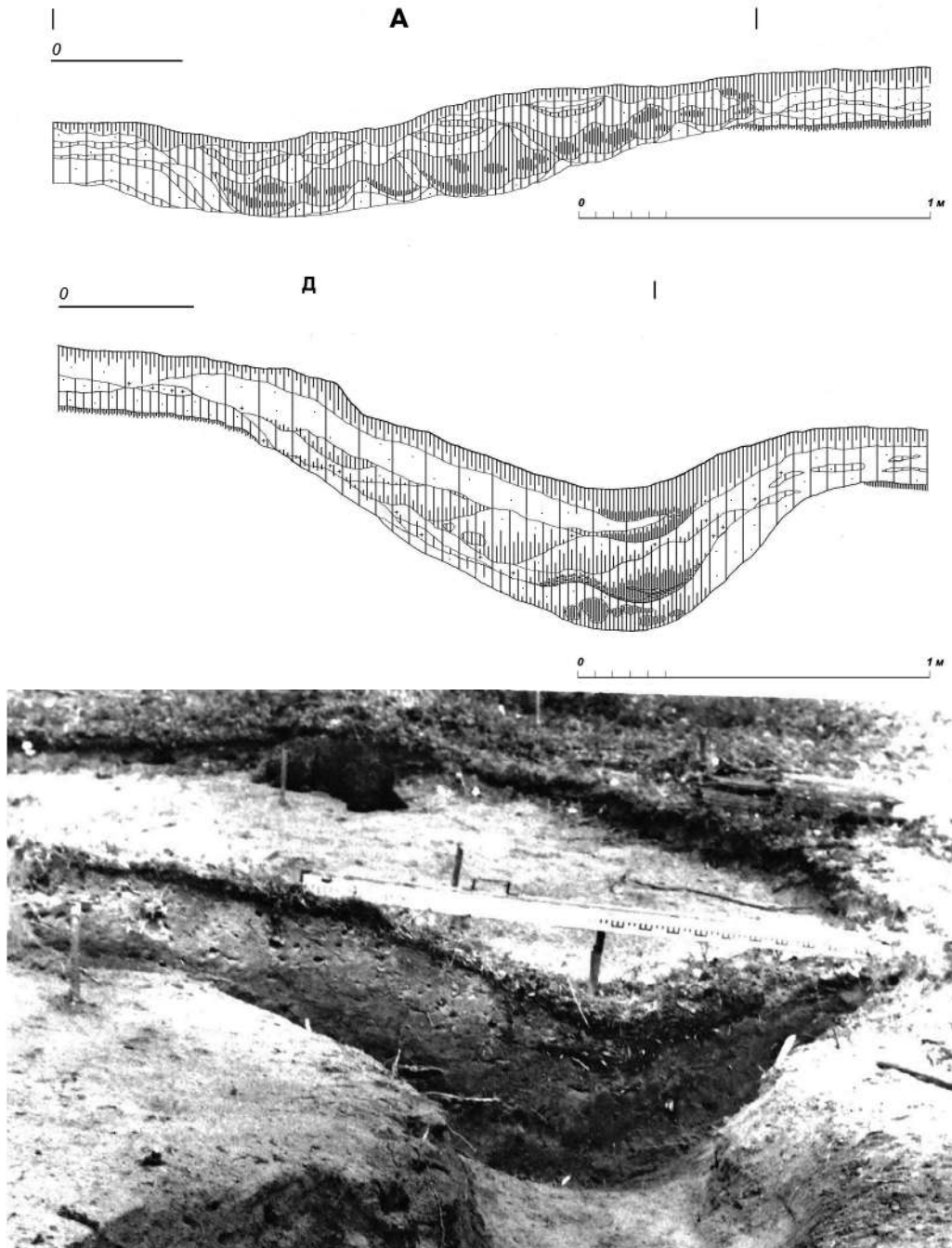
Рис. 4. Вскопление Шахново 3-1. Детали разрезов по оси 3 – В (западная и восточная части). Фото – деталь разреза вскопления Шахново 3-1 по оси 3 – В (восточная часть, вид с юга), фото автора
