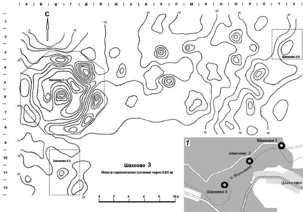
Рис. 1. Группа памятников Шахново-3. План в горизонталях (сечение через 0,05 м) и ситуационный план памятников близ дер. Шахново (1)
