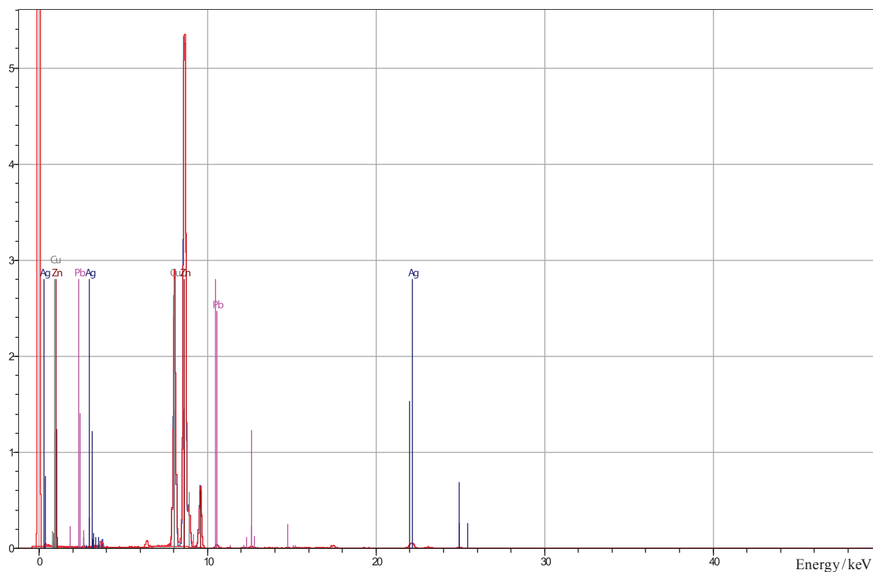
График 1. Элементный состав серебряного припоя в средокрестии
