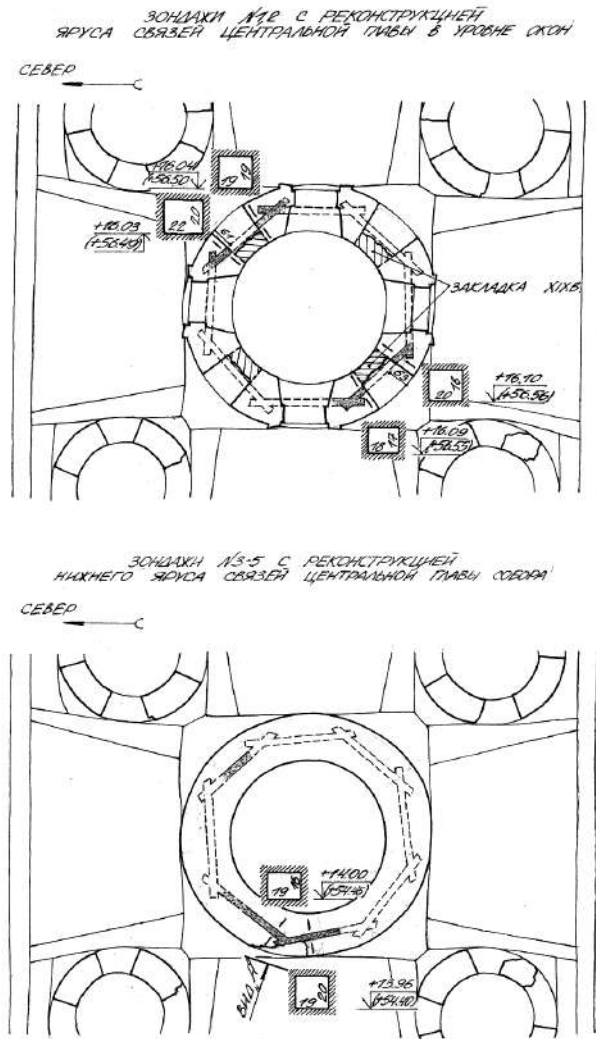
Рис. 2. Никольский собор в Новгороде. 1113 г. Реконструкция ярусов связей в центральном барабане. Чертеж Е. В. Скрипцовой. Архив ННРУ. Папка № 59
