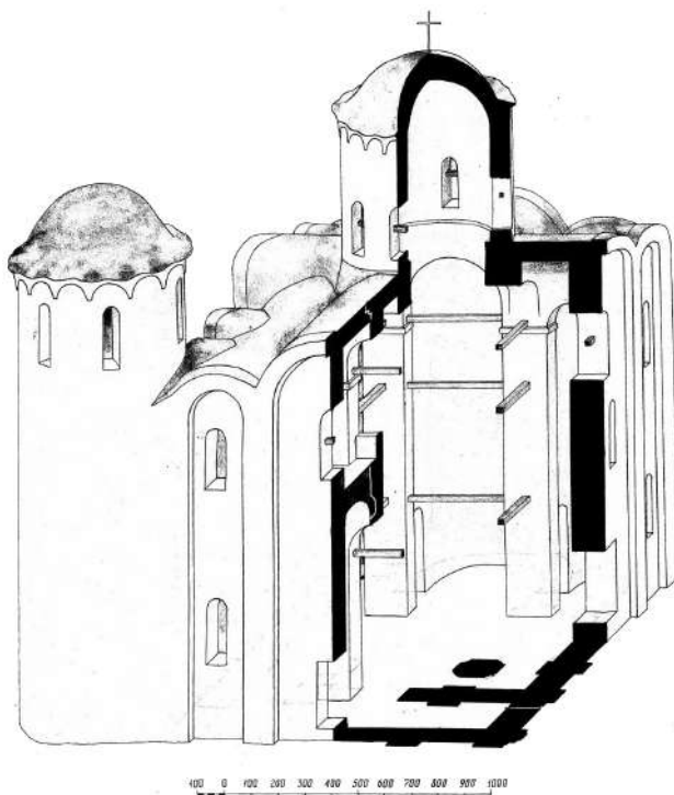
Рис. 1. Собор Рождества Богородицы Антониева монастыря в Новгороде. 1117–1119 гг. Реконструкция. Аксонометрия. Чертеж В. П. Огарковой. Архив ННРУ. Папка № 58
