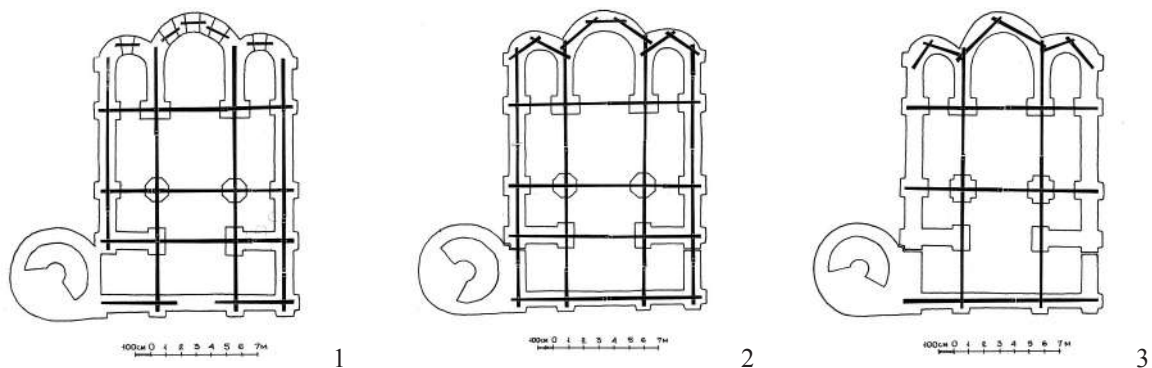
Рис. 3. Собор Рождества Богородицы Антониева монастыря в Новгороде. 1117–1119 гг. Реконструкция трех ярусов связей Л. Е. Красноречьева. По материалам чертежей А. С. Коробченко, А. А. Ковалева, Г. М. Кулаковой. Архив ННРУ. Папка № 589
