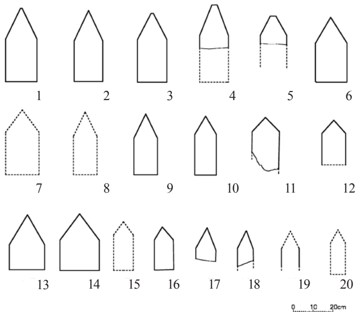
Рис. 3. Плинфы-«зубчики» XII–XIII вв.: 1–3 – Никольский собор на Дворище; 4–5 – Рождественский собор Антониева монастыря; 6 – Георгиевский собор Юрьева монастыря; 7 – церковь св. Климента в Ладогe; 8 – церковь Успения Богородицы в Старой Ладогe; 9–10 – церковь св. Георгия в Старой Ладогe; 11 – церковь Воскресения на Мячине; 12 – церковь св. Федора Стратилата на Щирковой ул.; 13–15 – церковь Спаса на Нередице; 16–18 – церковь св. Параскевы Пятницы на Торгу; 19 – церковь св. Михаила Архангела на Прусской улице; 20 – церковь Рождества Богородицы в Перыни. Рисунки автора
