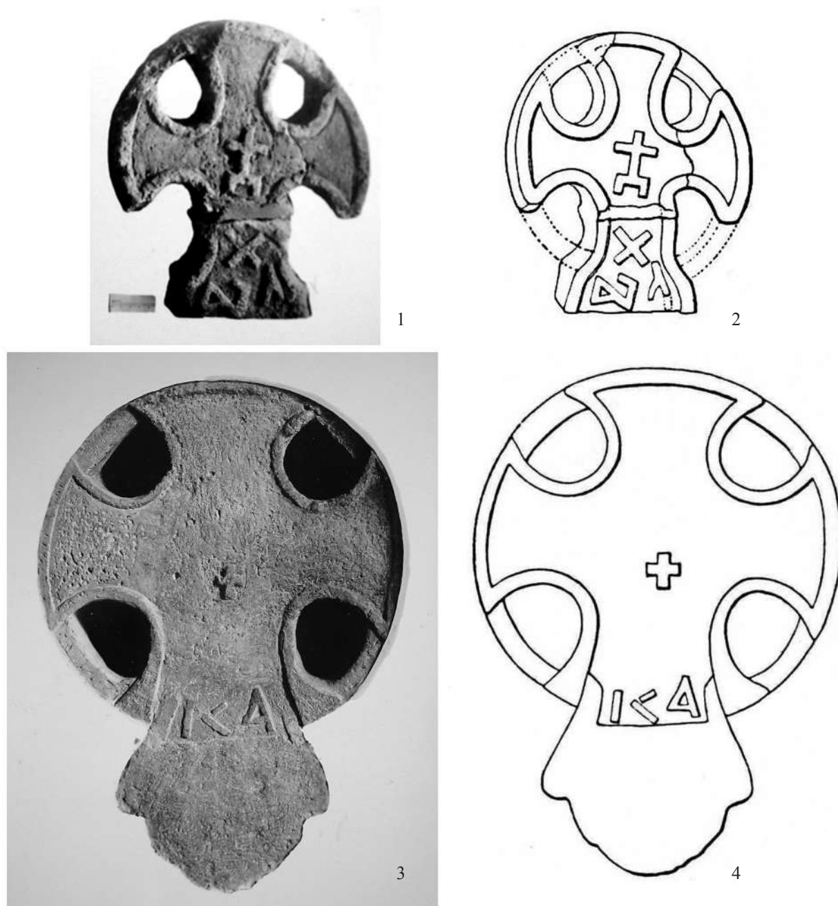
Рис. 2. Реставрированные кресты: 1 – Новгородский музей, 1903 г., ФО НА ИИМК РАН, Q.683. 17; 2 – по: Шляпкин 1906. Рис. 342; 3 – ФО НА ИИМК РАН, Q. 692. 5; 4 – по: Шляпкин 1906. Рис. 353 (Примечание: 1, 2 – к кресту без надписей вместо ножки присоединена правая боковая лопасть с монограммой ХЪ от другого креста; 3, 4 – новая верхняя часть креста «в круге» присоединена к ножке, ободок обрывается над монограммой; 3 – фотография креста подписана: «1896 г. Москва. Исторический музей. Новгородский зал. Каменный крест XIV в. Верхняя лопасть реставрирована»)
