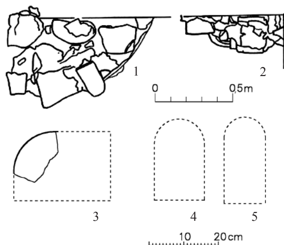
Рис. 6. Лекальная плинфа в кладках церкви св. Михаила Архангела на Прусской ул.: 1 – шурф № 2. План съехавшего блока кладки апсиды; 2 – шурф № 3. Фрагмент апсиды с полуколонкой; 3 – плинфа с полукруглым углом; 4–5 – плинфа с полукруглым тычком. 1–2 – Архив ННРУ. Папка 160; 3–5 – рисунки автора
