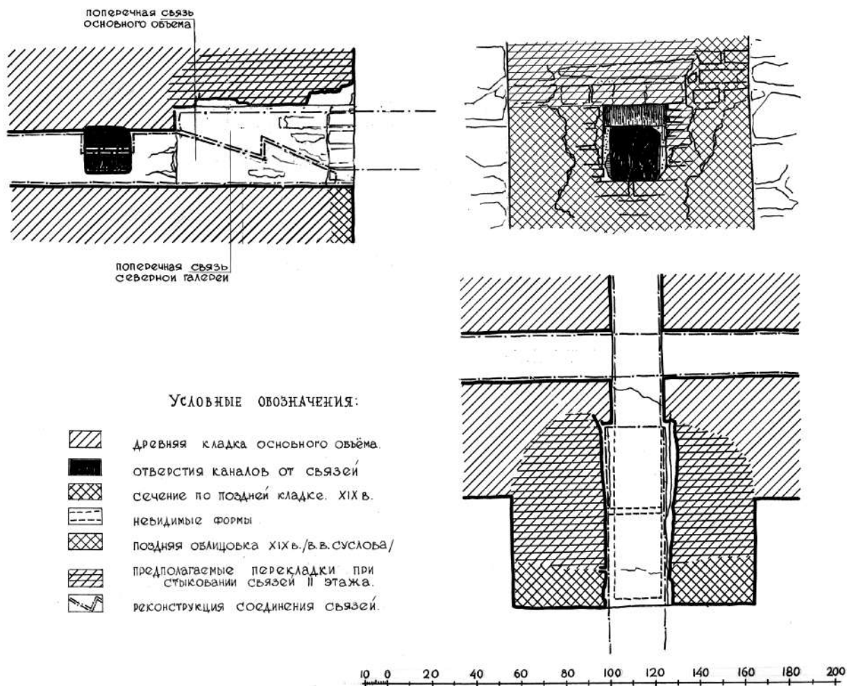
Рис. 4. Софийский собор в Новгороде. 1045–1050 гг. Соединение связей основного объема и второго этажа северной галереи. Чертеж Г. М. Штендера. Архив ННРУ. Папка № 1
