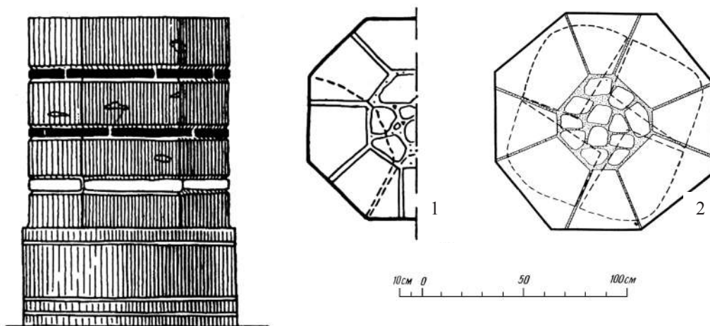
Рис. 2. Схема укладки плитки в восьмигранных столбах: 1 – София Новгородская. Фасад и план столба хор. Реконструкция Г. М. Штендера (по: Штендер 1974. Рис. 1); 2 – Десятинная церковь в Киеве (ремонт XI в.?). Реконструкция Г. Ю. Ивакина (по: Ивакин 1979. С. 121)
