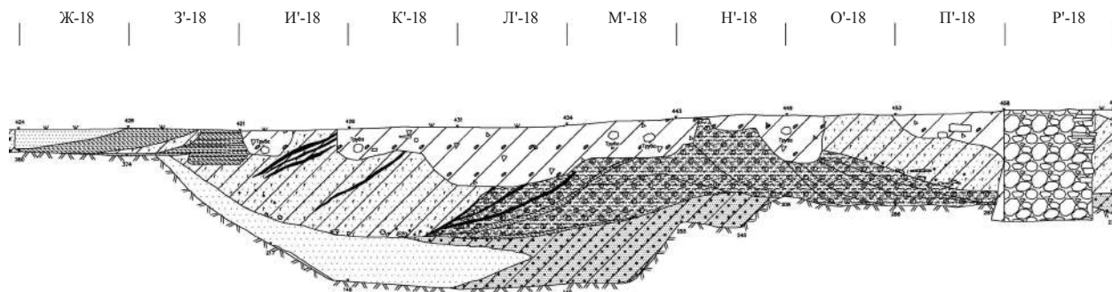
Рис. 3. Археологический контекст находки креста: стратиграфический разрез заполнения рва вблизи места находки. Авторы: П. Е. Сорокин, К. А. Михайлов, В. Д. Гукин
