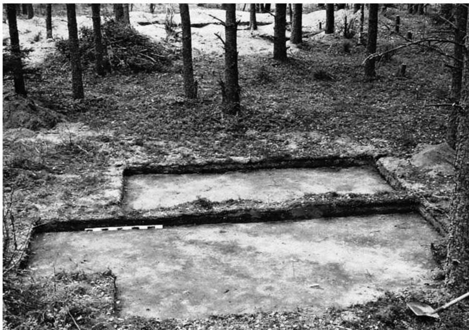
Рис. 5. Объекты Шахново 3-2 и Шахново 3-3: 1 – объект Шахново 3-2, план и разрез следов и остатков в южном раскопе; 2 – объект Шахново 3-3, план и разрез следов и остатков в восточном раскопе, Фото – объект Шахново 3-3. Общий вид с востока, фото автора
