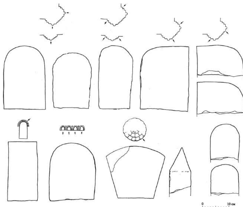
Рис. 5. Разновидности лекальной плинфы, примененной в кладках церкви св. Параскевы Пятницы на Торгу. Архив ННРУ. Папка 51. Инв. № 2264-2272
