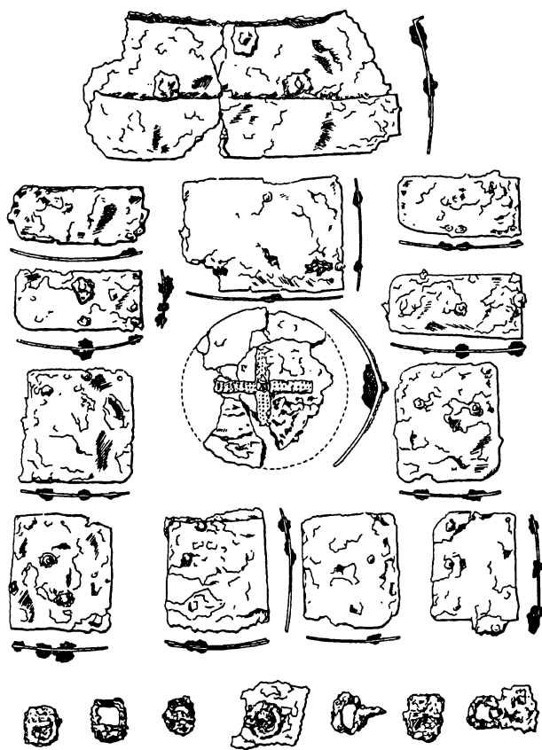
Пластинчатый доспех из раскопок в Довмантовом городе. Псков. XIII в. (По В. Д. Белецкому)
