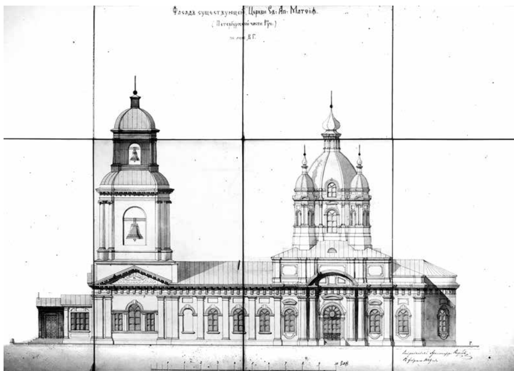
Матфеевская церковь, южный фасад, Санкт-Петербург. Чертеж архитектора Л. И. Карпова, 12 февраля 1889 г. (ФО. Отп. О.3623-4)
