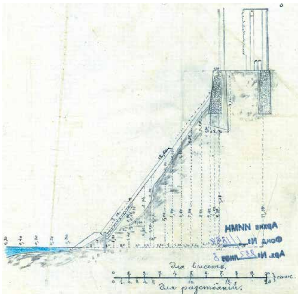
Схема устройства укрепляющей площадки под Коложской церковью, Гродно (РО. Ф. 1. Оп. 1-1894 г. Д. 233. Л. 8)
