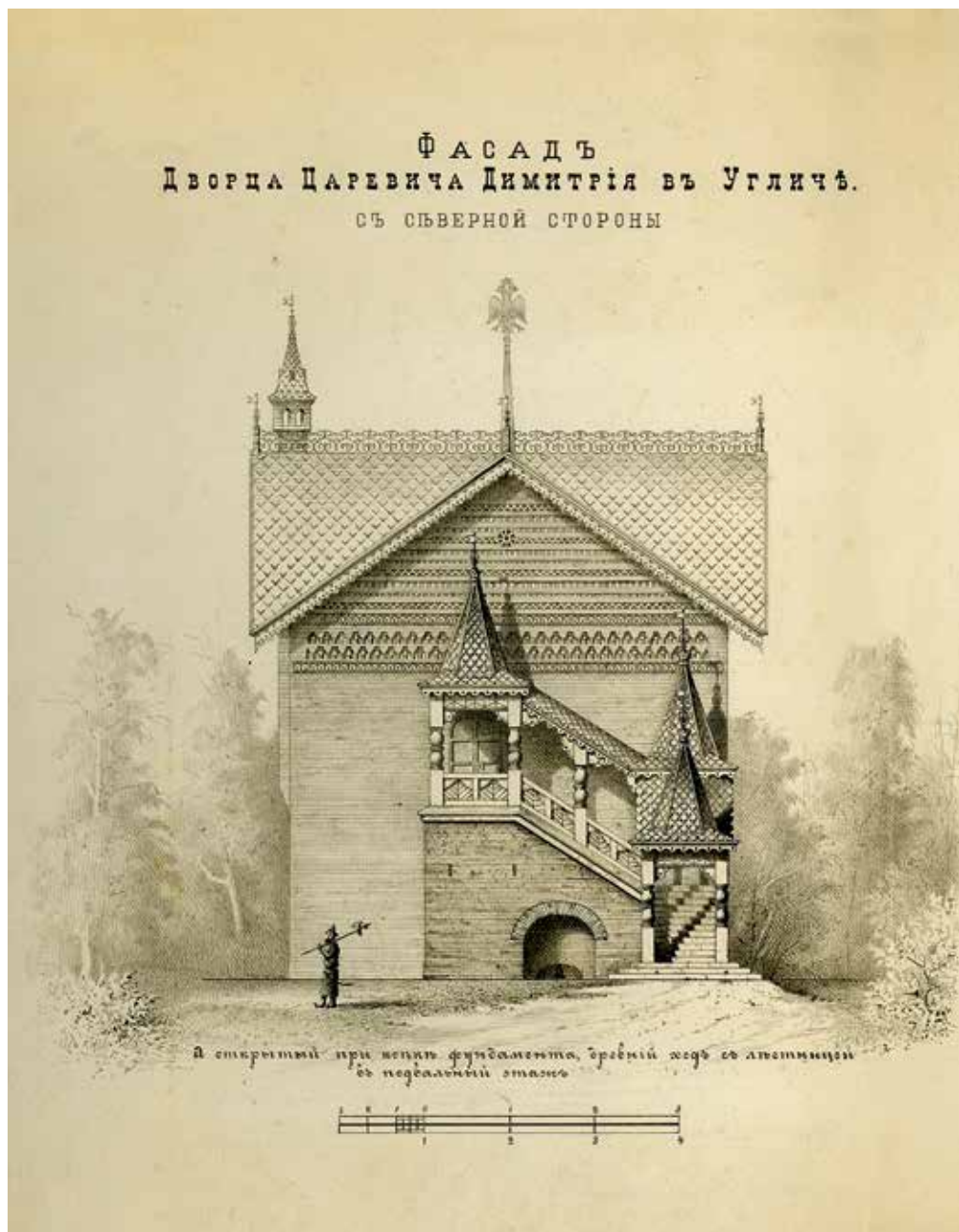
Северный фасад дворца царевича Дмитрия в Угличе. Эскизный проект И. А. Шлякова (РО. Ф. 1. Оп. 1-1888 г. Д. 41. Л. 162)
