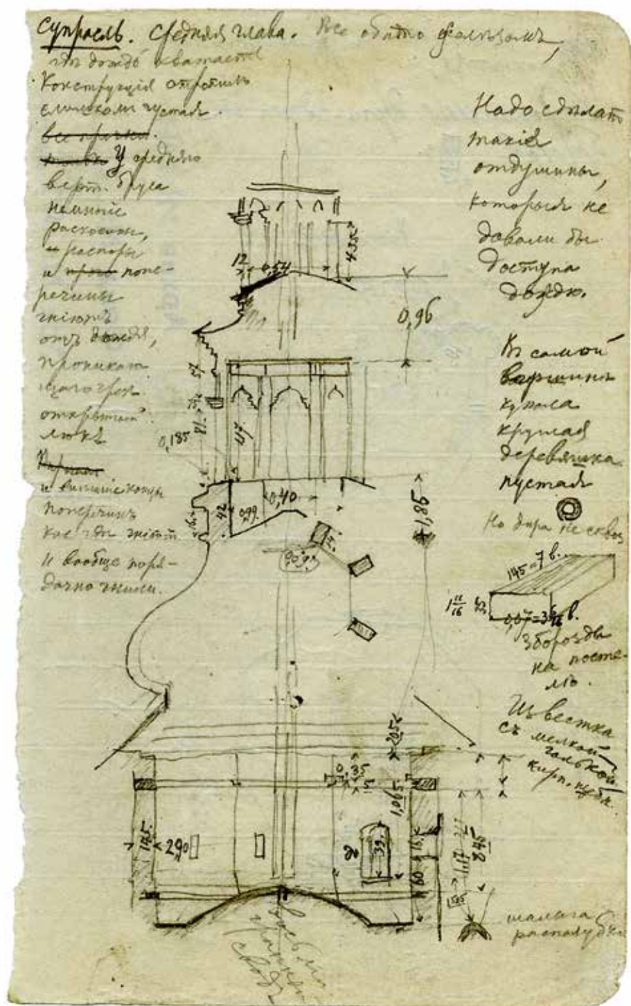
Разрез средней главы Благовещенской церкви Супрасльского монастыря с размерами и примечаниями. Рисунок П. П. Покрышкина, 1910 г. (?) (РО. Ф. 21. Оп. 1. Д. 543. Л. 2 об.)
