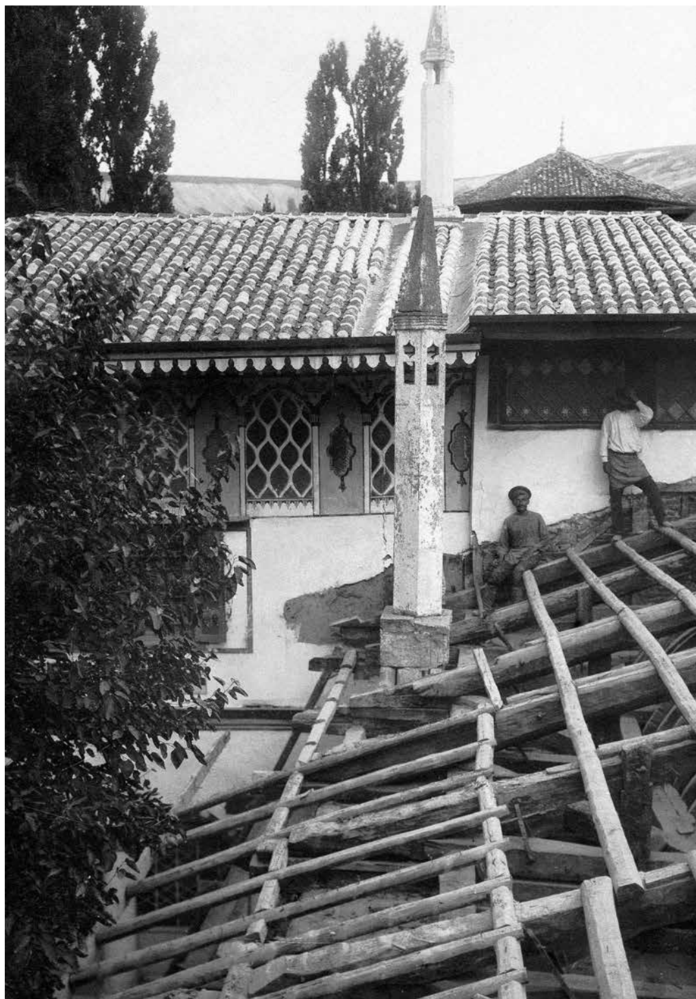
Ханский дворец, зал суда. Деталь конструкции крыши. Бахчисарай, Таврическая губерния. Фотография С. С. Некрасова, 1915 г. (ФО. Отп. О. 412-2233)
