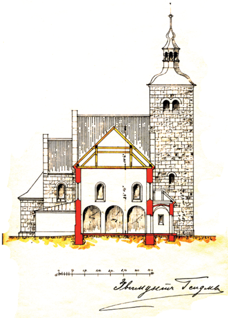
Чертеж поперечного разреза костела св. Николая, XIII в., Высоцице, Меховский уезд, Келецкая губерния (РО. Ф. 1. Оп. 1-1904. Д. 25. Л. 26)
