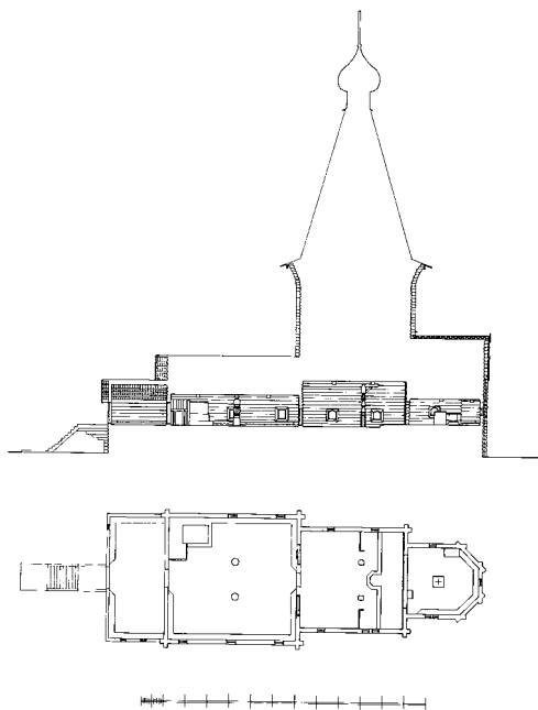
Петропавловская церковь в с. Пучуга, Вологодская губерния. Чертежи Д. В. Милеева (ФО. Нег. III 9934)
