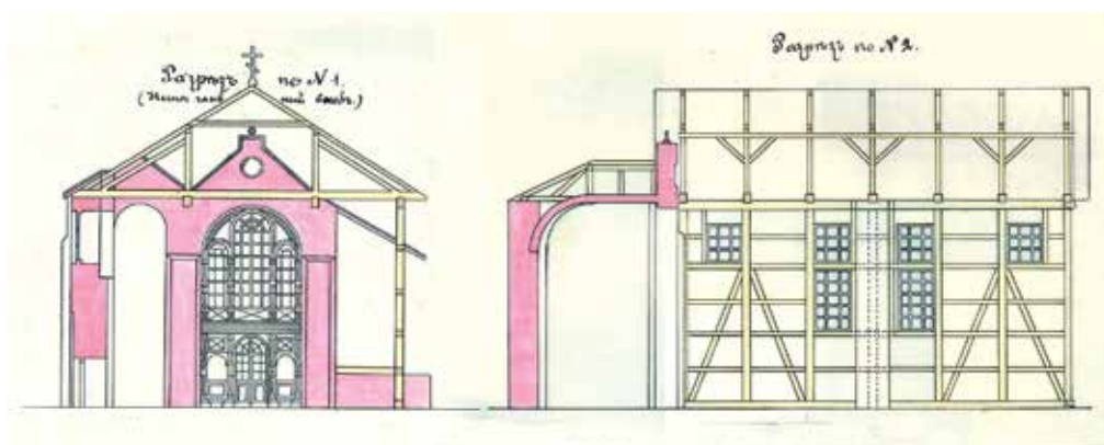
Проект деревянного покрытия и стен Коложской церкви, Гродно (РО. Ф. 1. Оп. 1-1894 г. Д. 233. Л. 14)
