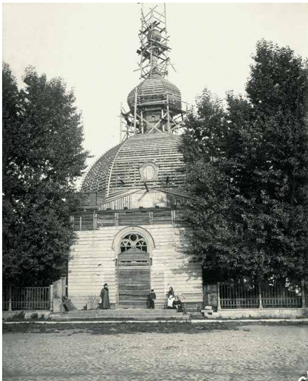
Троице-Петровский собор на Петербургской стороне, Санкт-Петербург. Реставрация после пожара 1913 г. (ФО. Отп. О.3602-14)
