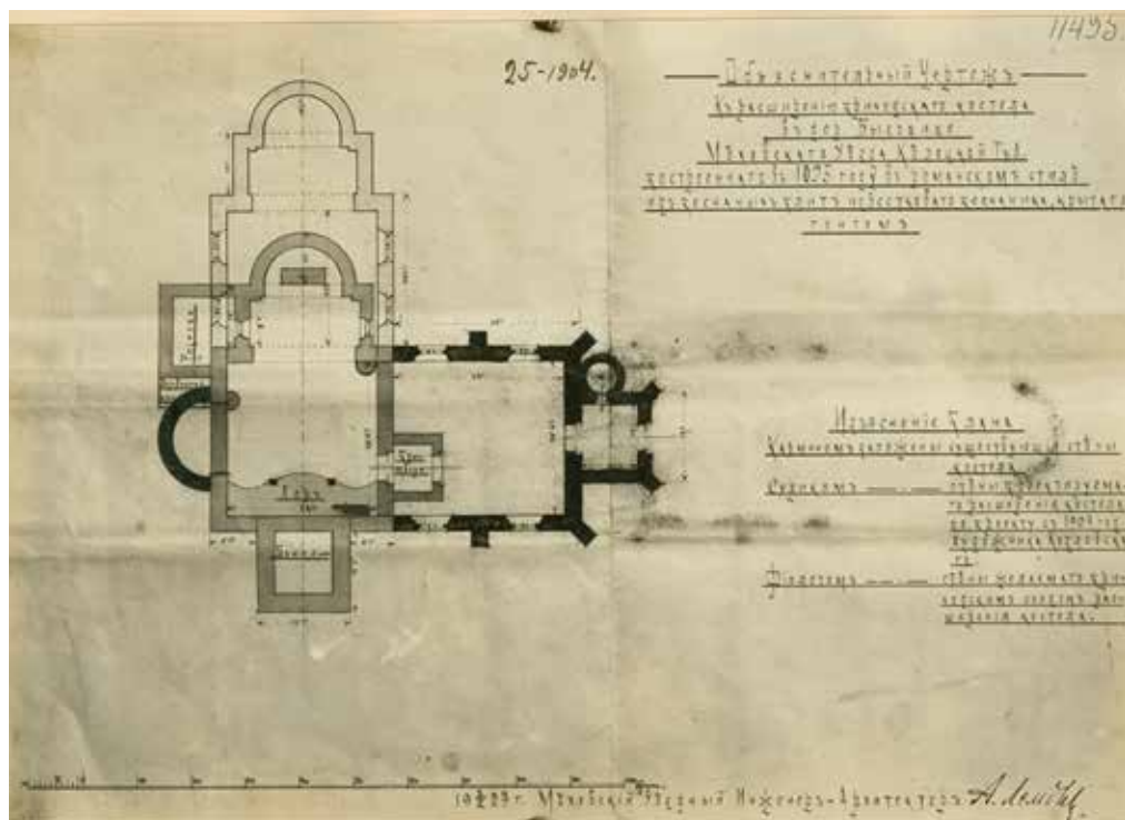
План переустройства и расширения романского костела св. Николая, XIII в., Высочице, Меховский уезд, Келецкая губерния (РО. Ф. 1. Оп. 1-1904. Д. 25. Л. 20)
