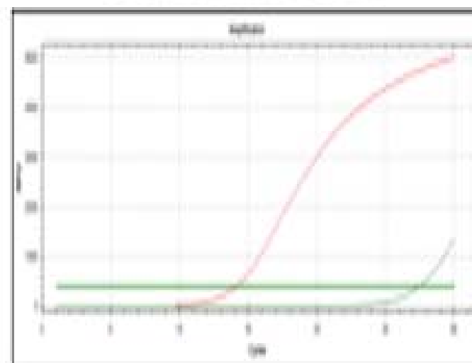
S. constellatus UCN96
