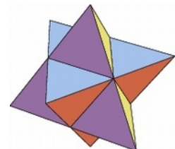
Octaèdre étoilé
