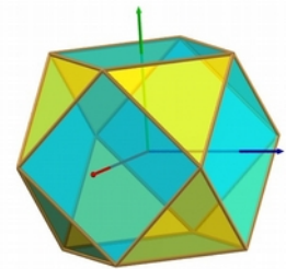
Cuboctaèdre
