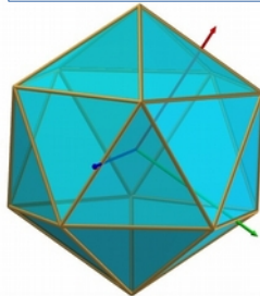
Icosaèdre
