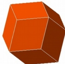
Dodecaèdre rhombique
