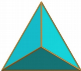
Tetraèdre
