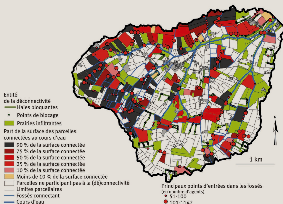
2 Cartographie des entités de la (dé)connectivité sur le bassin versant de Lingèvres (2014) – Reulier et al. , 2017.
