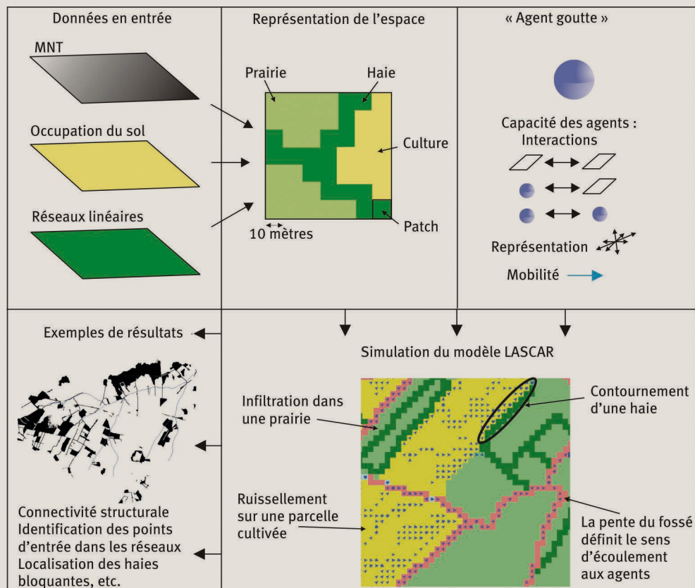
❶ Présentation simplifiée du modèle LASCAR (la bibliographie fournit les références nécessaires à la bonne compréhension du modèle).
