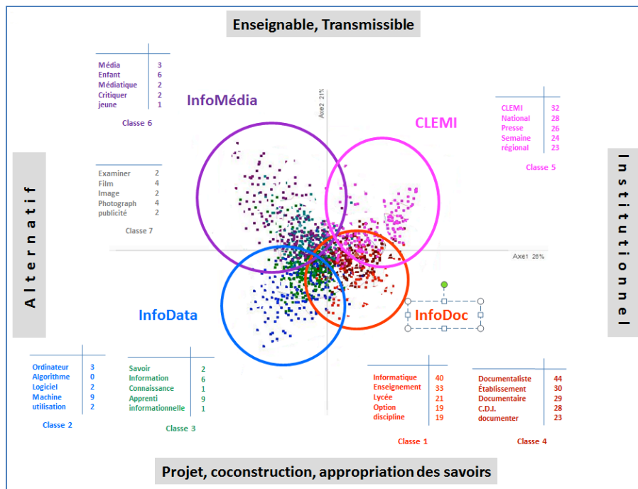
Figure 3. AFC étiquetée
