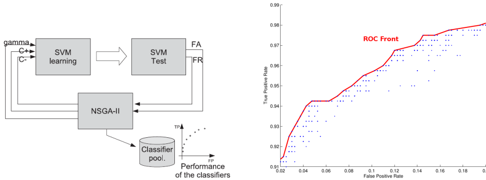
FIG. 1: Front ROC en classification binaire. Gauche : illustration de la méthode, utilisée avec des classifieurs de types SVM (tiré de Chatelain et al. (2010)); Droite : représentation du Front dans l'espace ROC qui permet de visualiser chaque classifieur via ses TVP ( i.e. 1-TFN) et TFP.
