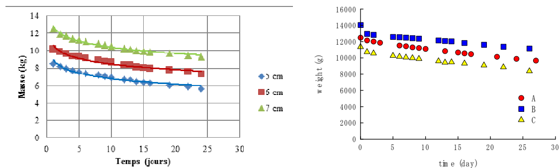
(a) Essais sur les sédiments d'Honfleur Epaisseurs de la couche de sédiments : 5, 6 7 cm.
